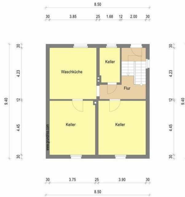
Kellergeschoss
