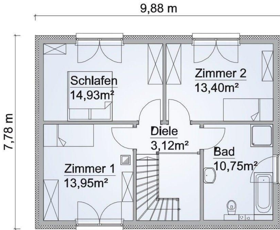
SH 122 S Variante A (OG)
